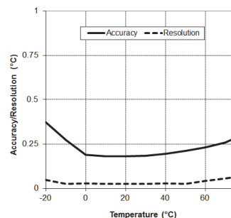
Grafik A: Temperaturgenauigkeit und Auflösung
